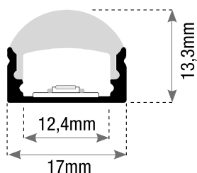
KPRI40G-2413 (INCASSO)
