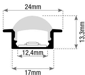
KPRS40G-1713 (SUPERFICIE)
