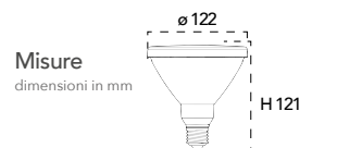
Lampada LED classe A+ E27 PAR38 18W 230V
