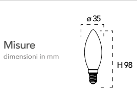
Lampada LED classe A++ 6W 230V
