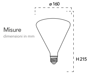
Lampada LED decorativa classe B 8W 230V
