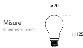
Lampada LED filamento classe A+ 16W 230V
