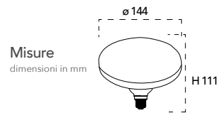
Lampada LED classe A+ E27 DSL 15W 230V
