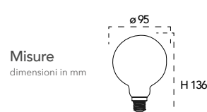
Lampada LED filamento classe A++ 8W 230V
