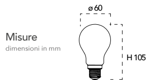
Lampada LED classe A+ 8W 230V
