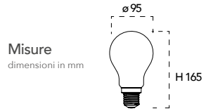
Lampada LED filamento classe A+ 23W 230V
