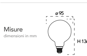
Lampada LED filamento classe A++ 8W 230V
