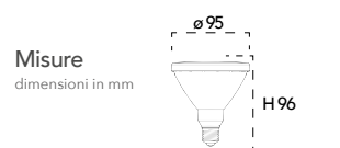
Lampada LED classe A+ E27 PAR30 12W 230V
